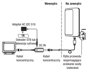
Rys. 4: Eksploatacja za pomocą zasilacza
