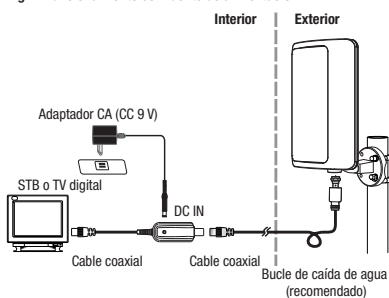
Fig. 4: Funcionamiento con fuente de alimentación
