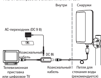
Рис. 4: Режим работы с блоком питания от сети
