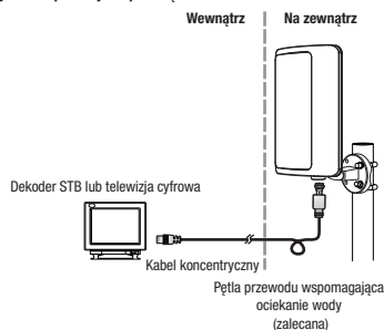
Rys. 3: Eksploatacja za pomocą dekodera STB
